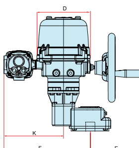
Приводы ОМEx10-12
