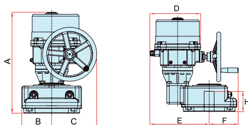
Привод OM 10-12
