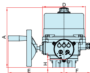
Привод OM 2-9
