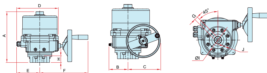
Привод OM 2-9
