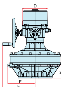
Привод OM 13-15
