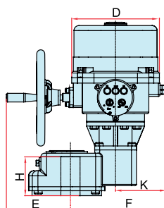
Привод OM 2-9
