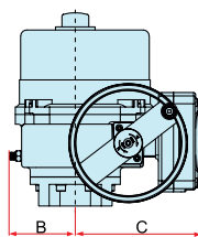
Привод OM 2-9
